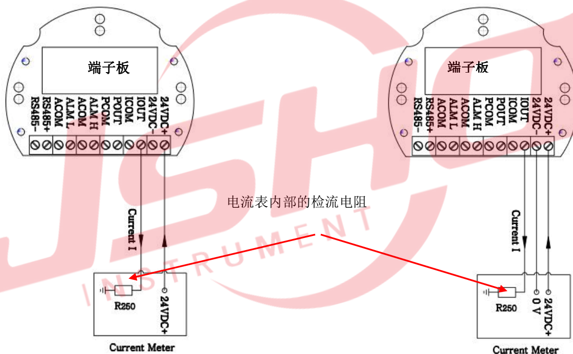
二线制接线图
